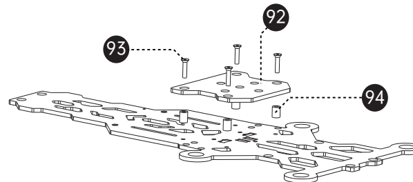
手持云台板套件 Gimbal carbon plate Kit
