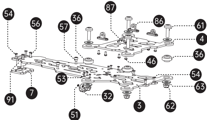
机身部分 (顶部) Main body frame: Top plate
