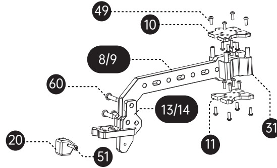
机臂部分 Frame Arm
