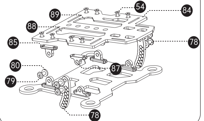
标准相机套件 Universal camera Kit
