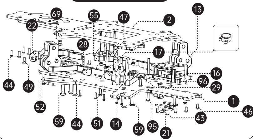
机身部分 (底部) Main body frame: Bottom plate
