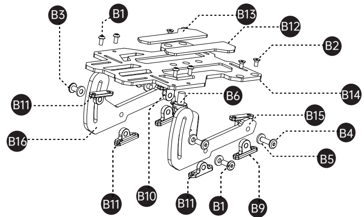
标准相机套件 Universal camera Kit
