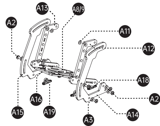
RED 相机套件 RED camera Kit
