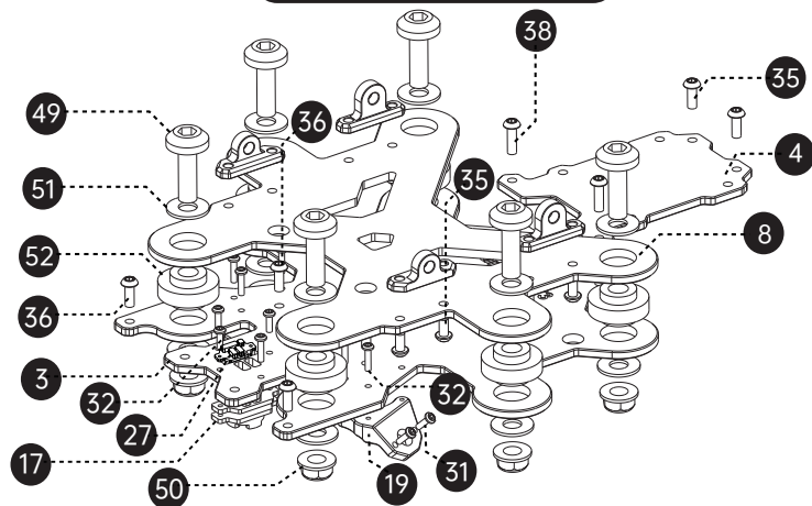
机身部分（顶板） Main body frame: Top plate
