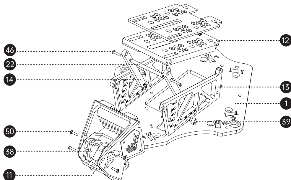
DJI O4版本安装示意图 DJI O4 Version Assembly diagram
